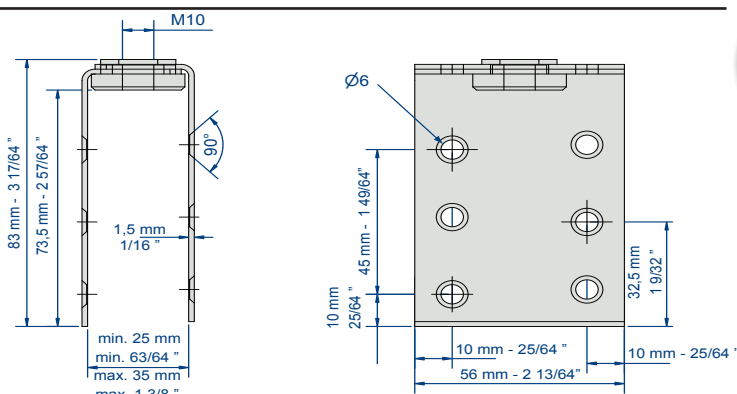
Apron set 0031
