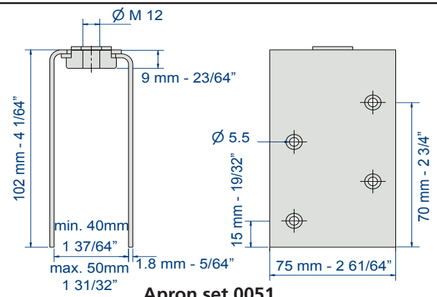
Apron set 0051
