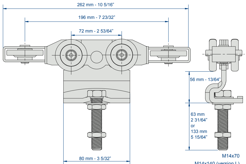
Hanger 9242 SE
